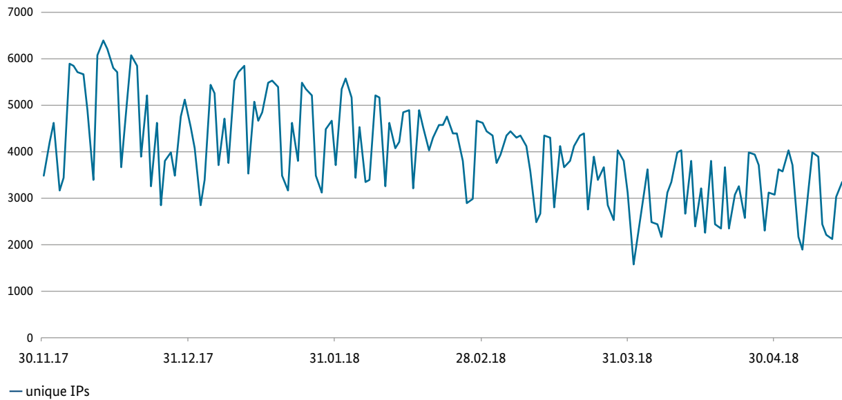
Abbildung 10.2 Infizierte Systeme
